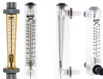
Flujómetro (Rotámetro)
